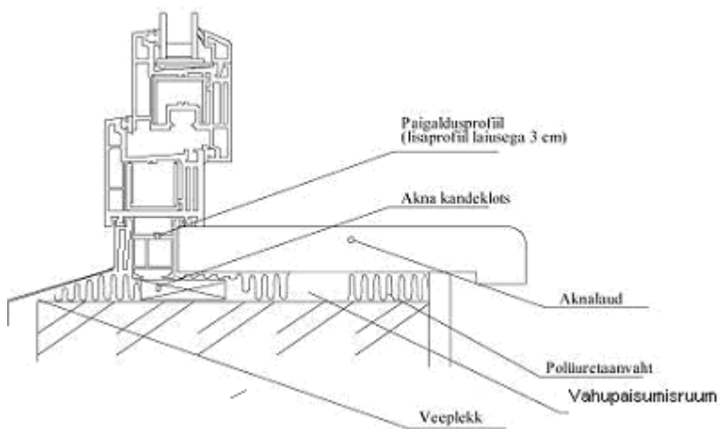
Joonis 10 . Aknalaua ja veepleki paigaldamine
